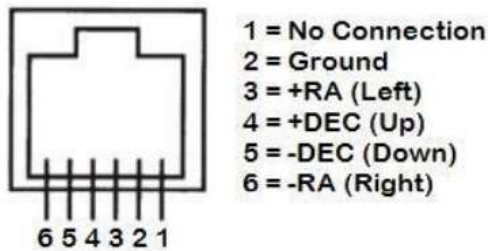
Pinout port ST-4 EQStarPRO
